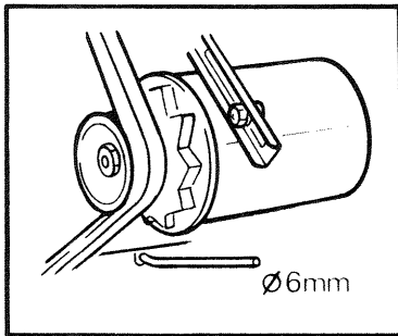
1) Stab in Bohrung für statische Zündeneinstellung.
